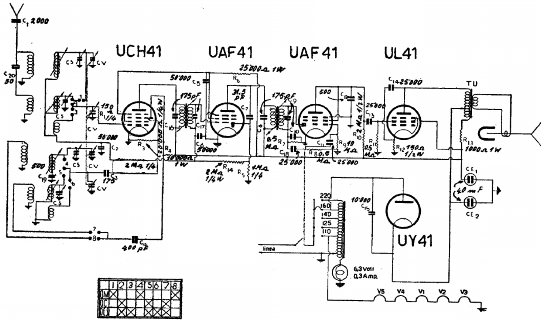
INCAR - Modd. VZ 507-508 - Onde medie e due corte. Potenza d'uscita 2 watt. Consumo 45 watt.
